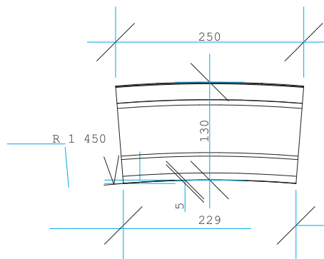
Декоративный элемент R3 коллекция «Тиволи» (Tivoli) Коды 735-х3 – 739-х3
