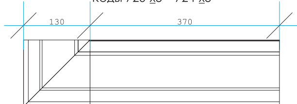
Декоративный элемент OL коллекция «Тиволи» (Tivoli) Коды 720-х3 – 724-х3
