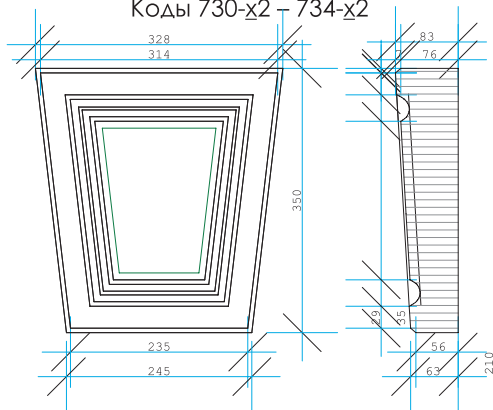
Варианты декорирования оконного проема
