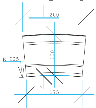
Декоративный элемент R2 коллекция «Тиволи» (Tivoli) Коды 735-х2 – 739-х2
