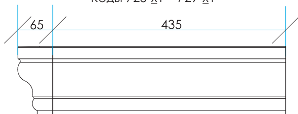
Декоративный элемент PL коллекция «Тиволи» (Tivoli) Коды 725-х1 – 729-х1
