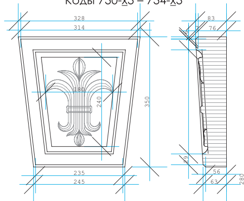
Декоративный элемент Z3 коллекция «Тиволи» (Tivoli) – замковый камень Коды 730-х3 – 734-х3
