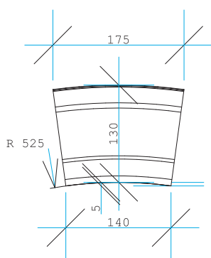
Декоративный элемент R1 коллекция «Тиволи» (Tivoli) Коды 735-х1 – 739-х1
