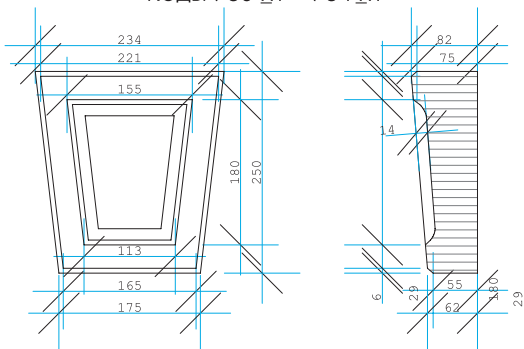
Декоративный элемент Z2 коллекция «Тиволи» (Tivoli) – замковый камень Коды 730-х2 – 734-х2
